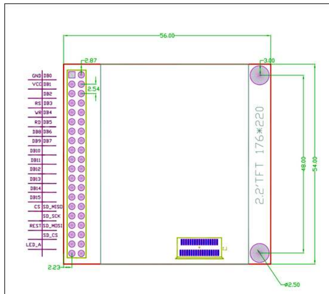
Рис.2 Установочные размеры
